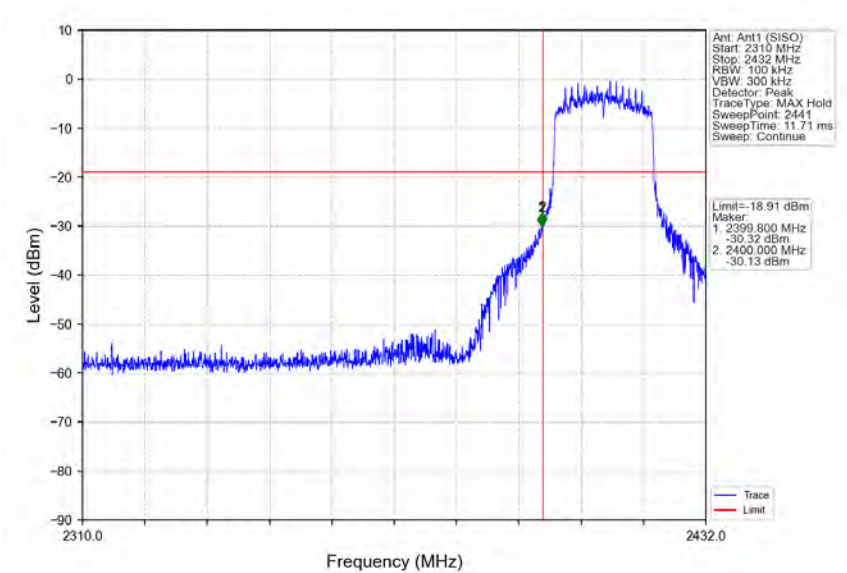
802.11ax(HEW20)_LCH_2412MHz_RU242_Left_Ant1 (SISO)_NTNV
