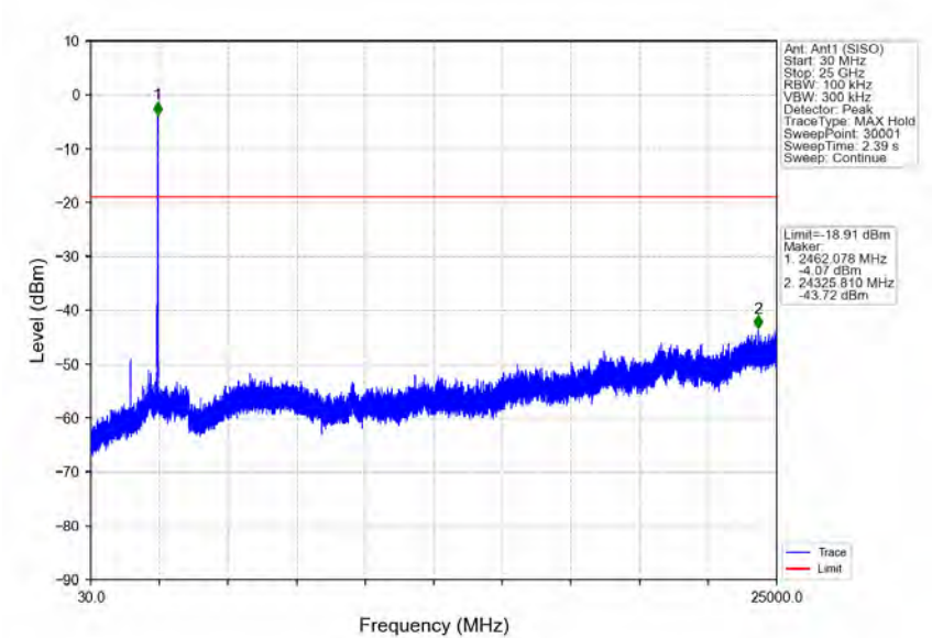
802.11ax(HEW20) HCH 2462MHz RU242 Left Ant1 (SISO) NTNV
