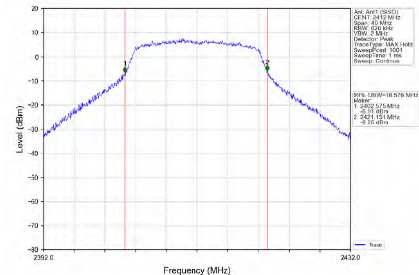
802.11g LCH 2412MHz Ant1 (SISO) NTN
