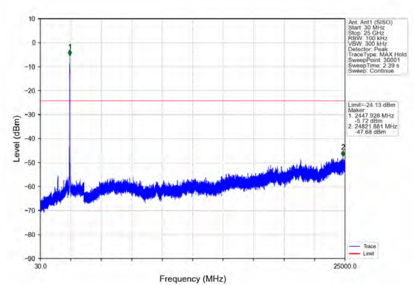
802.11ax(HEW40) MCH 2437MHz RU484 Left Ant1 (SISO) NTNV
