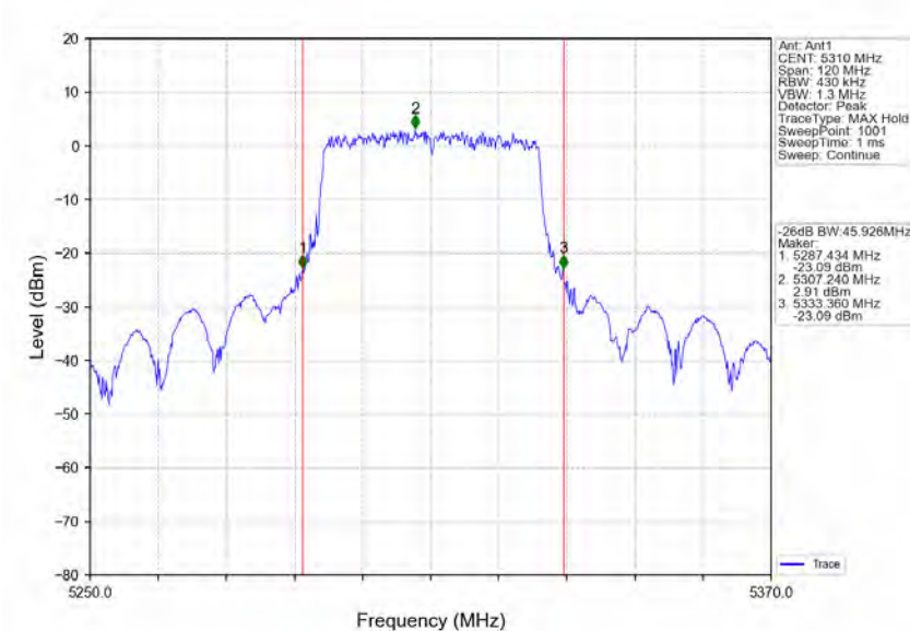
802.11ax(HEW40) HCH 5310MHz RU484 Left Ant1 NTNv
