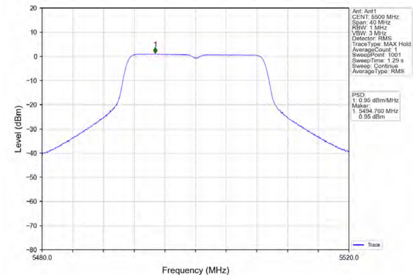
802.11ac(VHT20)_LCH_5500MHz_Ant1_NTNV
