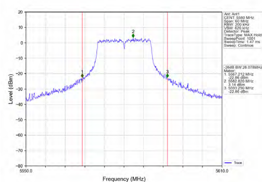
802.11a MCH 5580MHz Ant1 NTNV
