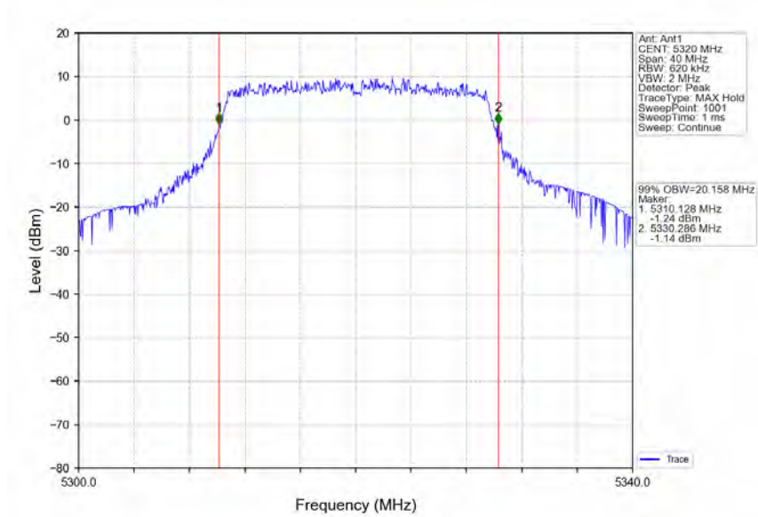
802.11ax(HEW20) HCH 5320MHz RU242 Left Ant1 NTNv
