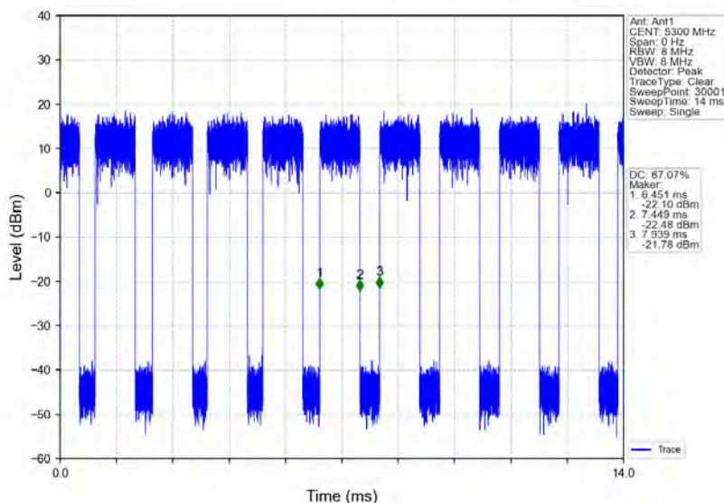
802.11ax(HEW20) MCH 5300MHz RU242 Left Ant1 NTNv
