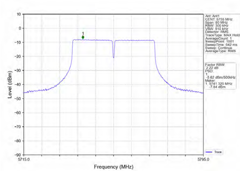
802.11ac(VHT40)_LCH_5755MHz_Ant1_NTNV
