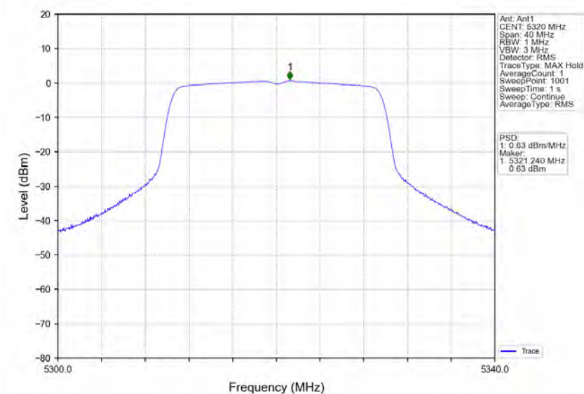
802.11ax(HEW20)_HCH_5320MHz_RU242_Left_Ant1_NTNV
