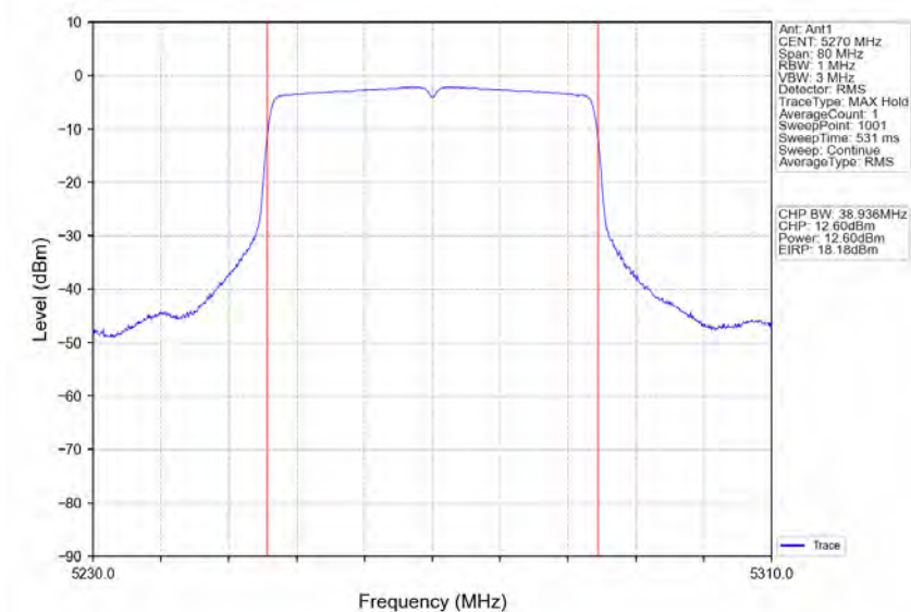
802.11ax(HEW40)_LCH_5270MHz_RU484_Left_Ant1_NTNV
