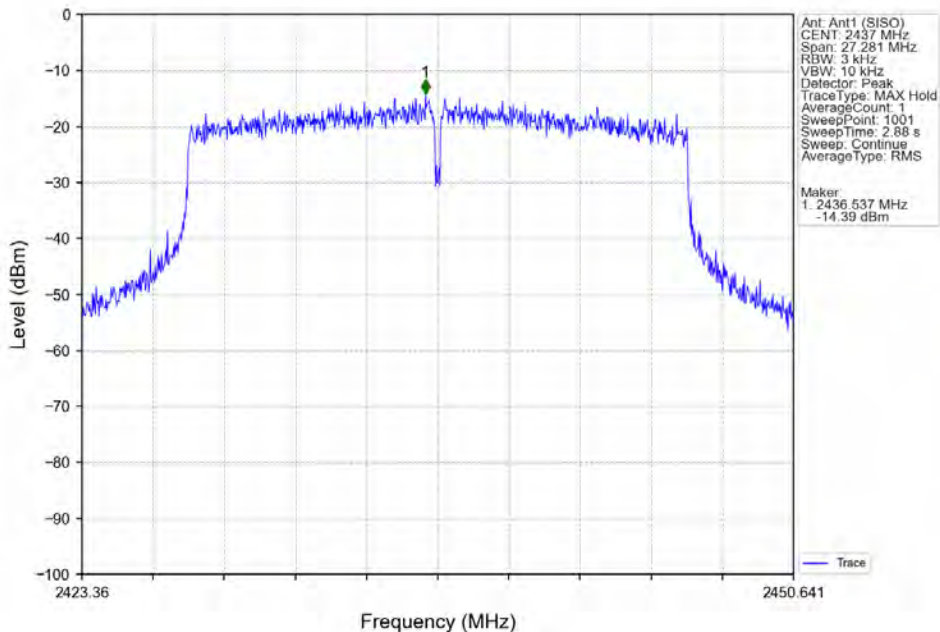
802.11ax(HE20)_MCH_2437MHz_RU242_Left_Ant1 (SISO)_NTNV
