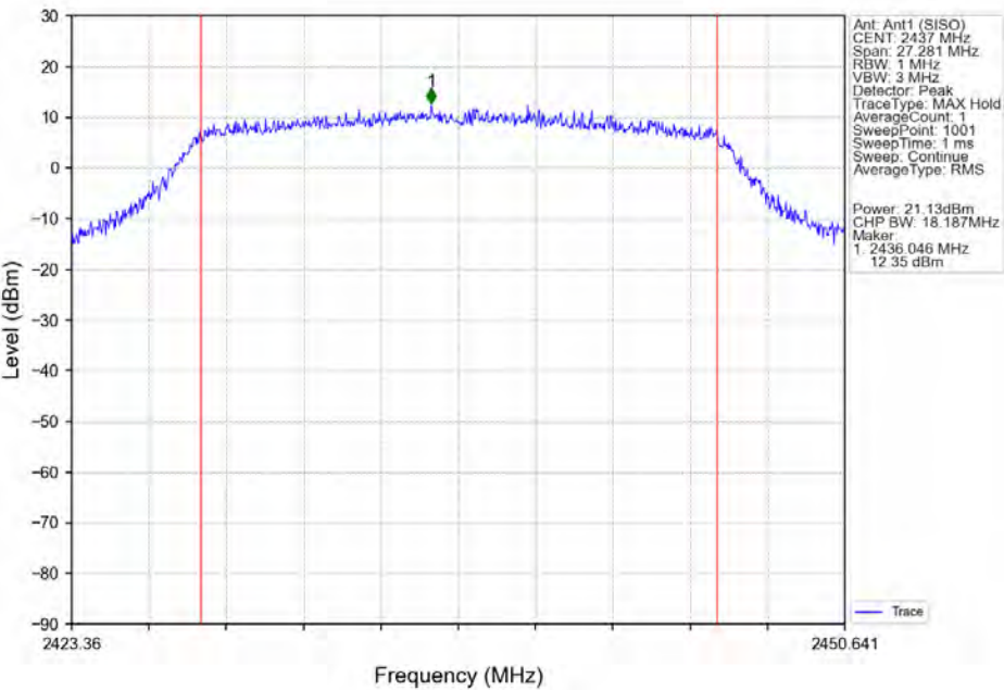
802.11ax(HE20)_MCH_2437MHz_RU242_Left_Ant1 (SISO)_NTNV
