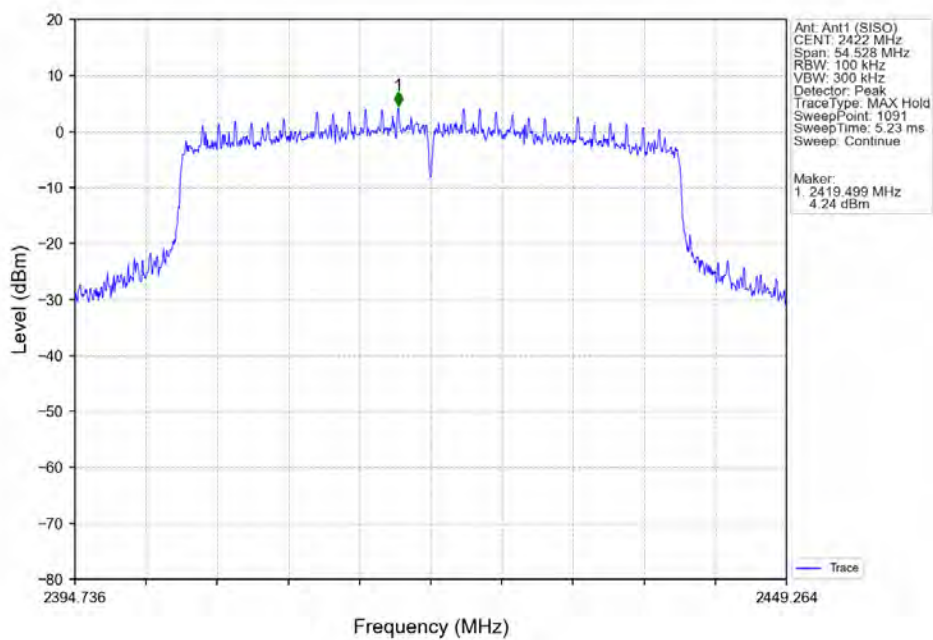
802.11ax(HE40)_LCH_2422MHz_RU484_Left_Ant1 (SISO)_NTNV
