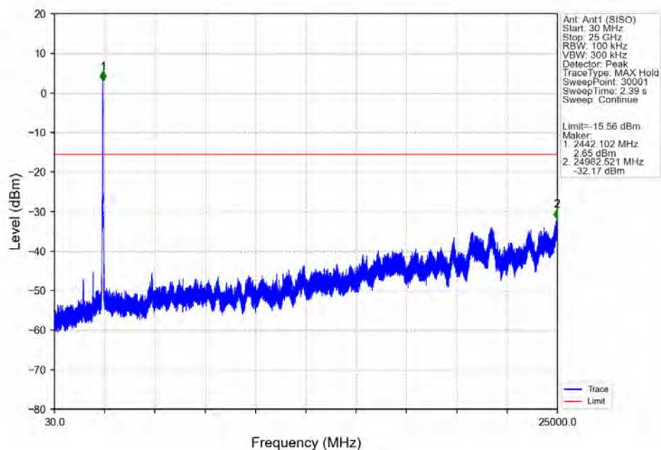
802.11ax(HE40)_MCH_2437MHz_RU484_Left_Ant1 (SISO)_NTNV
