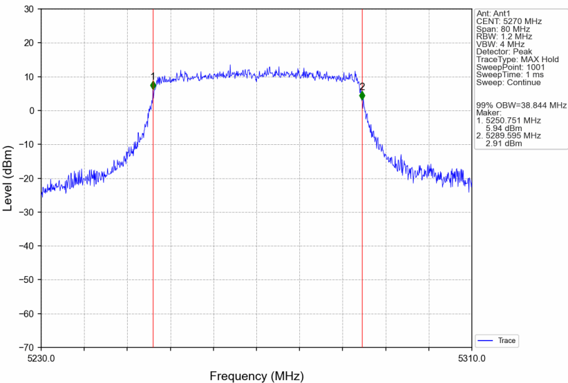
802.11ax(HE40)_LCH_5270MHz_RU484_Left_Ant1_NTNV
