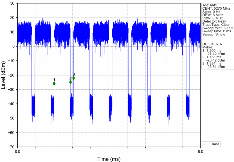
802.11ax(HE40)_LCH_5270MHz_RU484_Left_Ant1_NTNV
