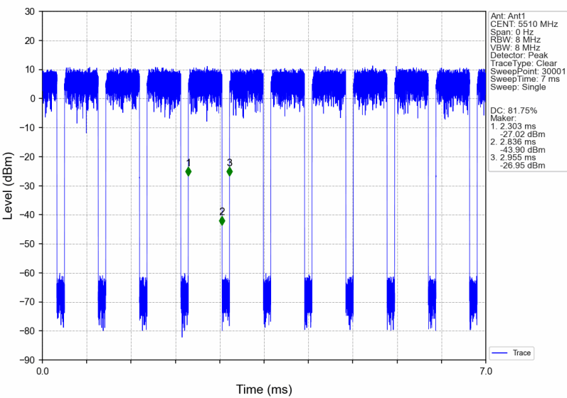
802.11ax(HE40)_LCH_5510MHz_RU484_Left_Ant1_NTNV
