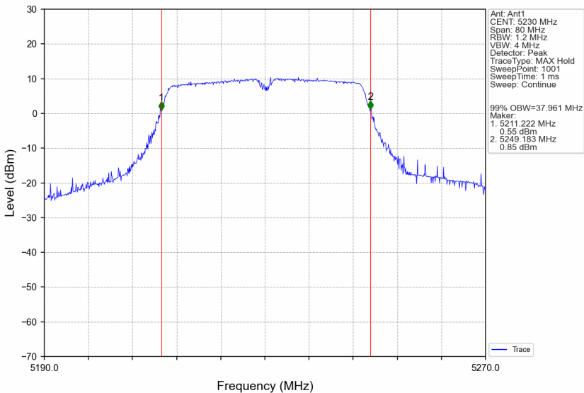
802.11ac(VHT40)_HCH_5230MHz_Ant1_NTNV
