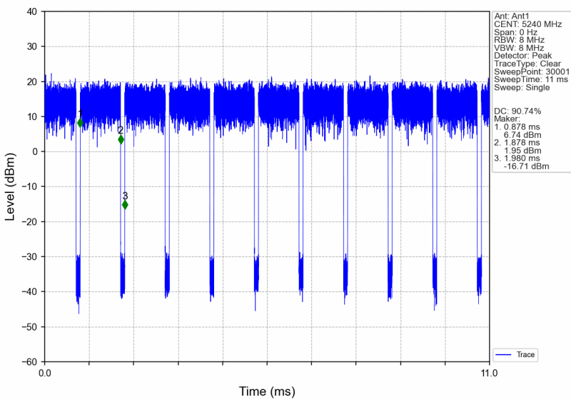
802.11ax(HE20)_HCH_5240MHz_RU242_Left_Ant1_NTNV
