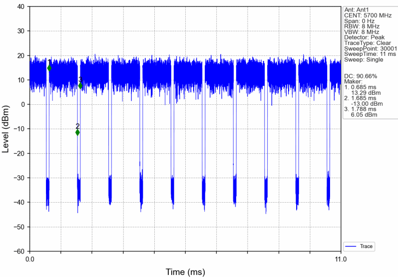
802.11ax(HE20)_HCH_5700MHz_RU242_Left_Ant1_NTNV
