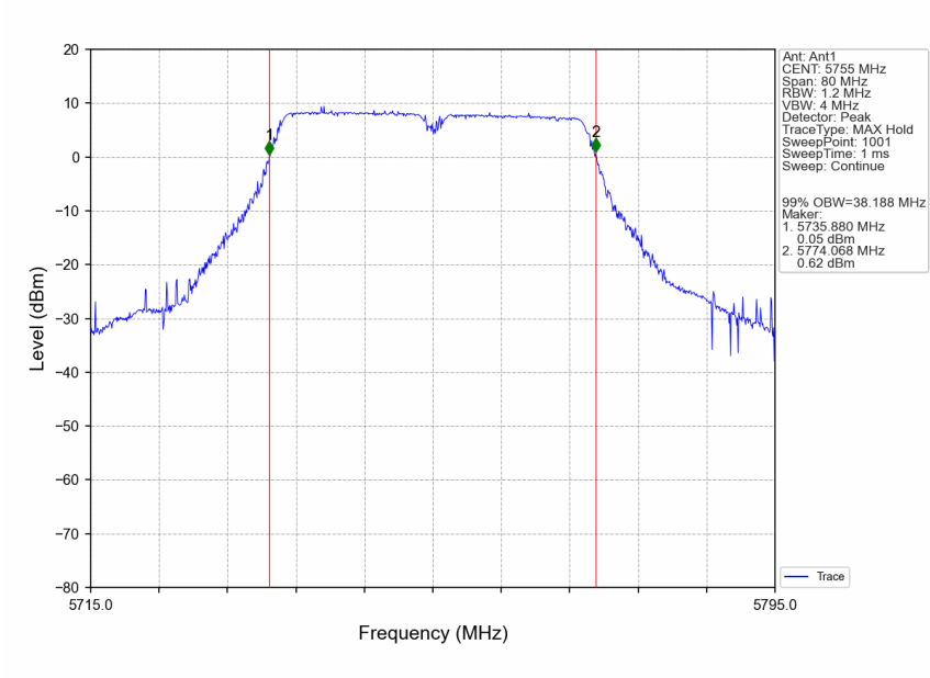
802.11ac(VHT40)_LCH_5755MHz_Ant1_NTNV
