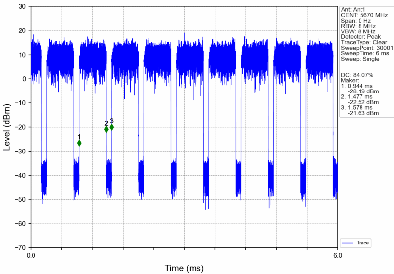
802.11ax(HE40)_HCH_5670MHz_RU484_Left_Ant1_NTNV
