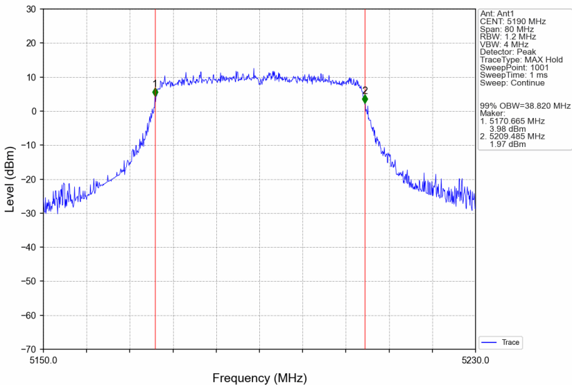
802.11ax(HE40)_LCH_5190MHz_RU484_Left_Ant1_NTNV
