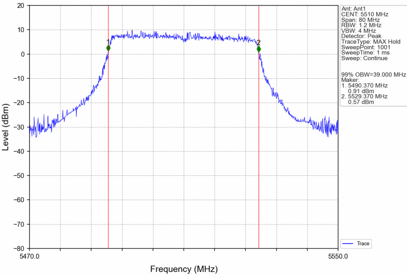
802.11ax(HE40)_LCH_5510MHz_RU484_Left_Ant1_NTNV
