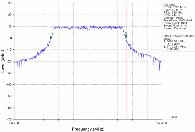
802.11ax(HE20)_HCH_5700MHz_RU242_Left_Ant1_NTNV
