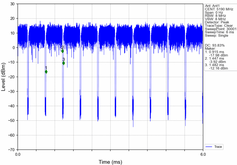
802.11ax(HE40)_LCH_5190MHz_RU484_Left_Ant1_NTNV
