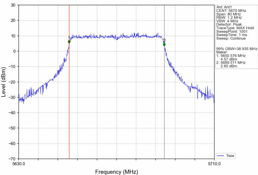
802.11ax(HE40)_HCH_5670MHz_RU484_Left_Ant1_NTNV
