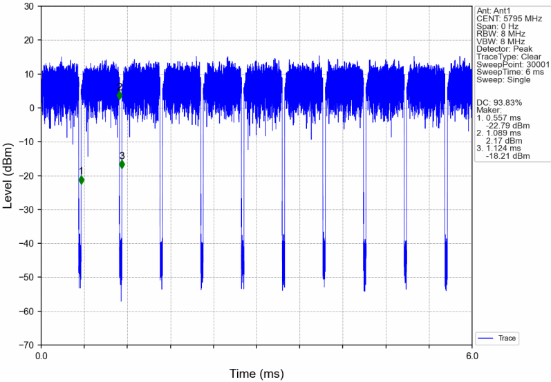
802.11ax(HE40)_HCH_5795MHz_RU484_Left_Ant1_NTNV
