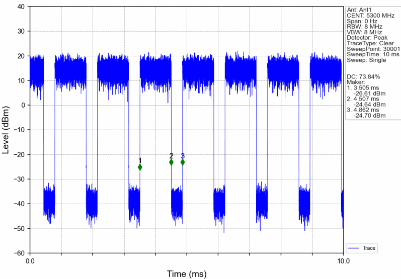
802.11ax(HE20)_MCH_5300MHz_RU242_Left_Ant1_NTNV
