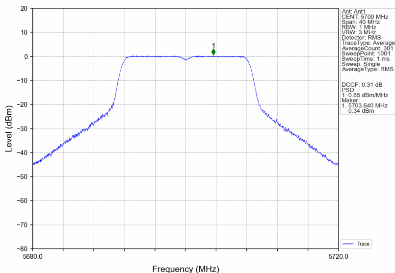
802.11a HCH 5700MHz Ant1 NTNV
