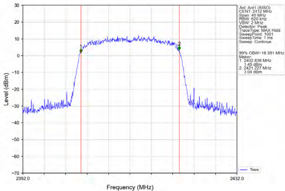
802.11ax(HE20) LCH 2412MHz SU / Ant1 (SISO) NTNV
