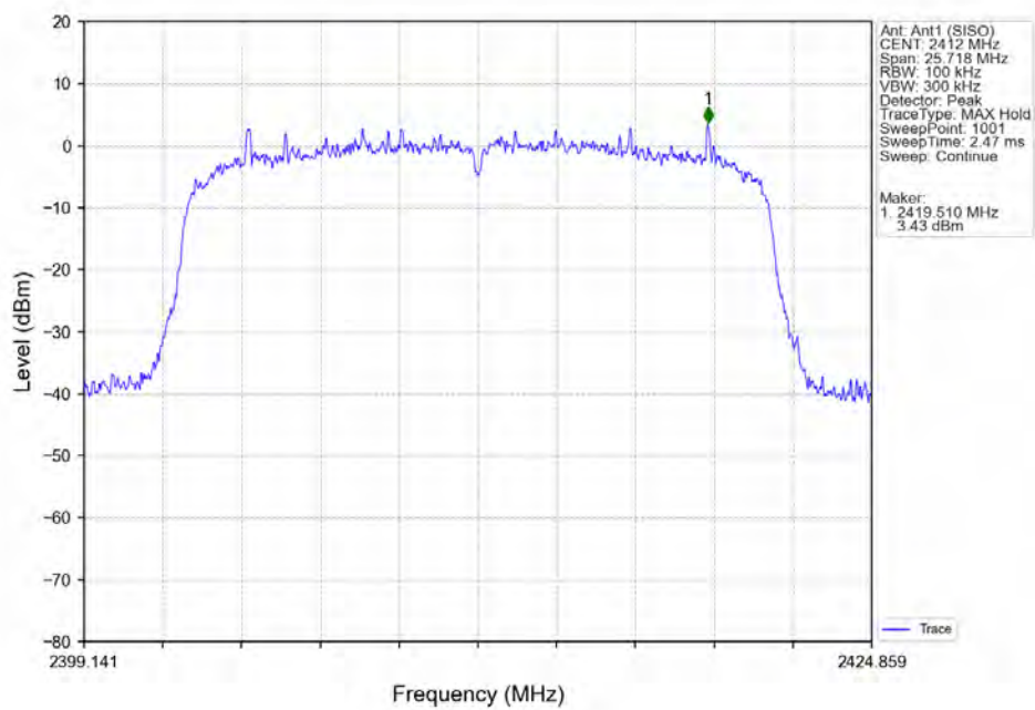
802.11ax(HE20) LCH 2412MHz SU / Ant1 (SISO) NTN
