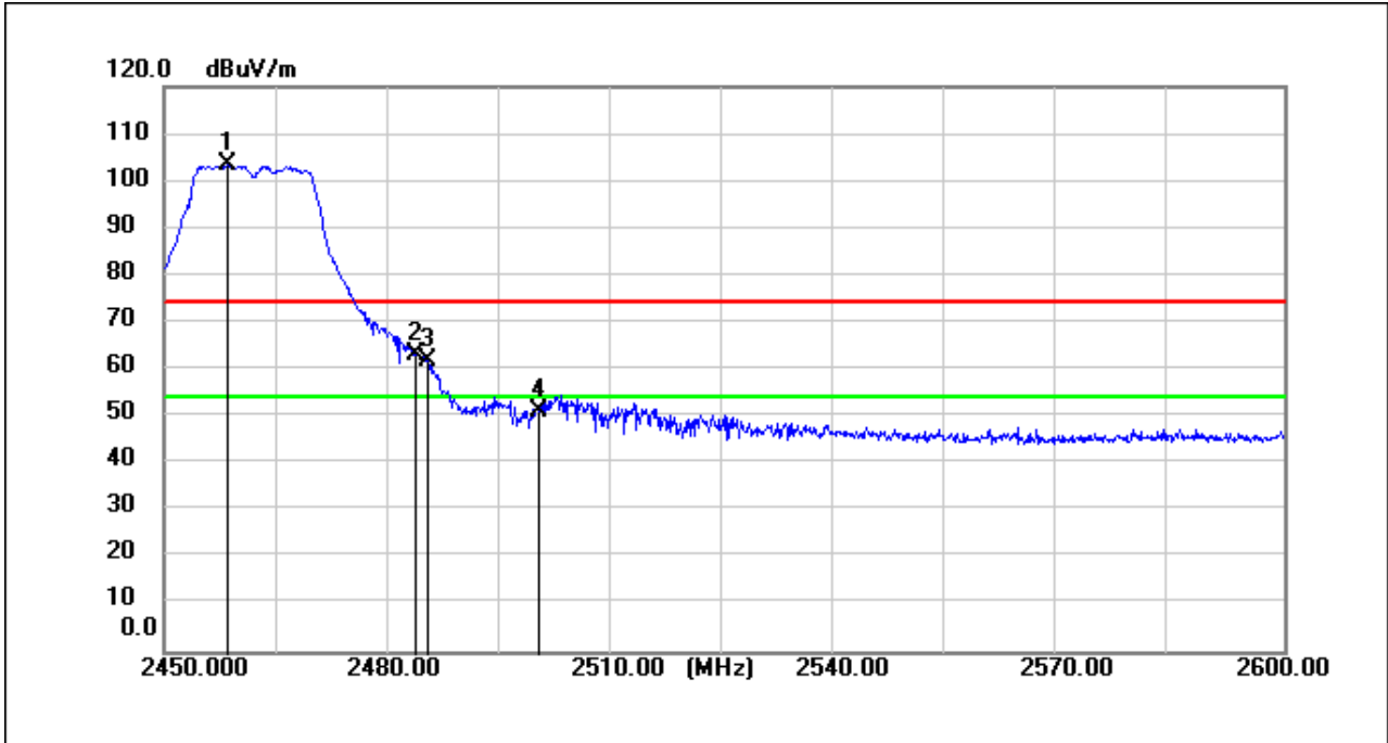
11n(HT20)_TX_CH_11_Vertical_Peak
