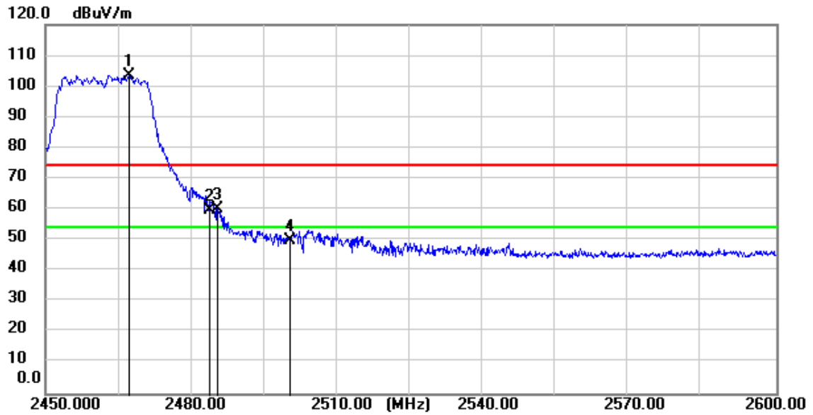
11(HE20)_TX_CH_11_Horizontal_Peak
