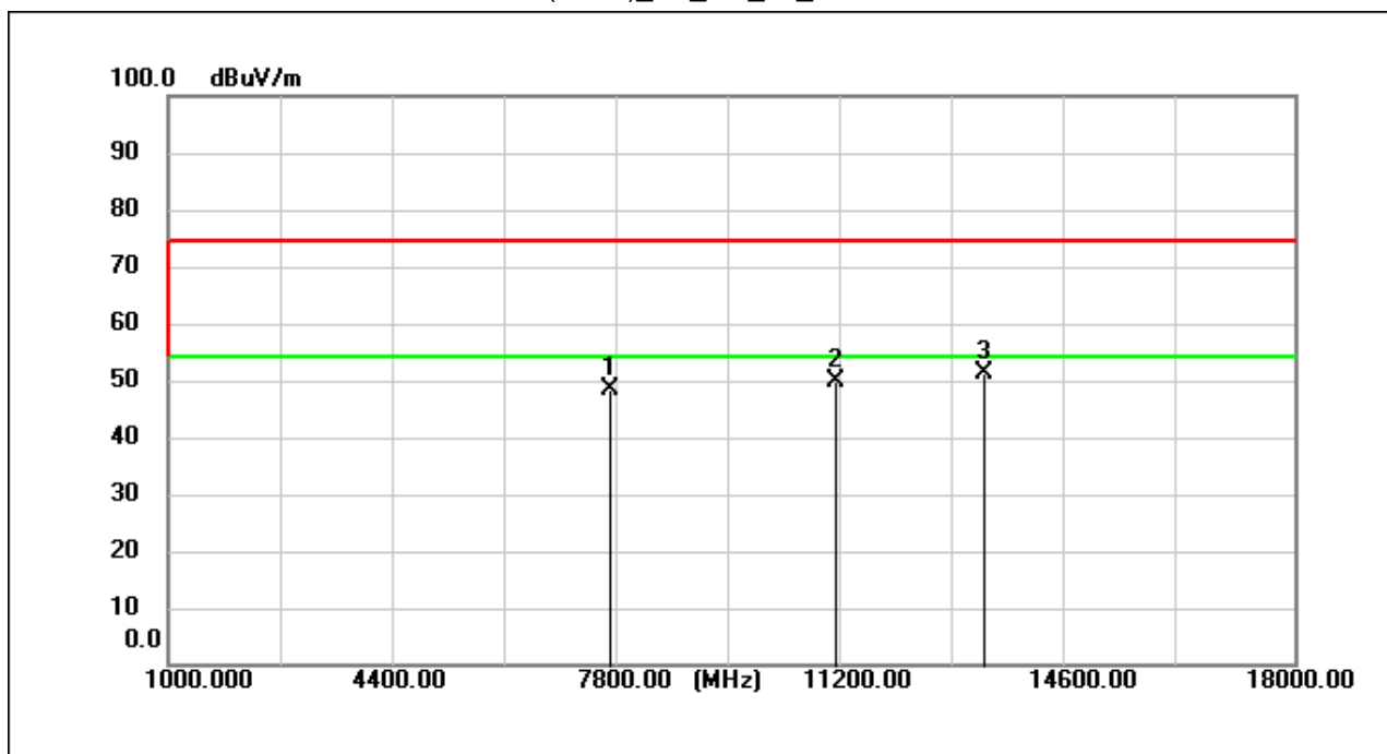
11n(HT20)_TX_CH_01_Vertical
