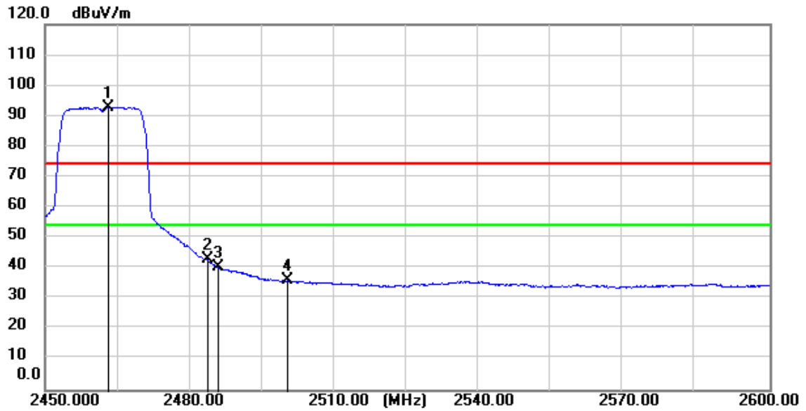
11n(HT20)_TX_CH_11_Horizontal_Average
