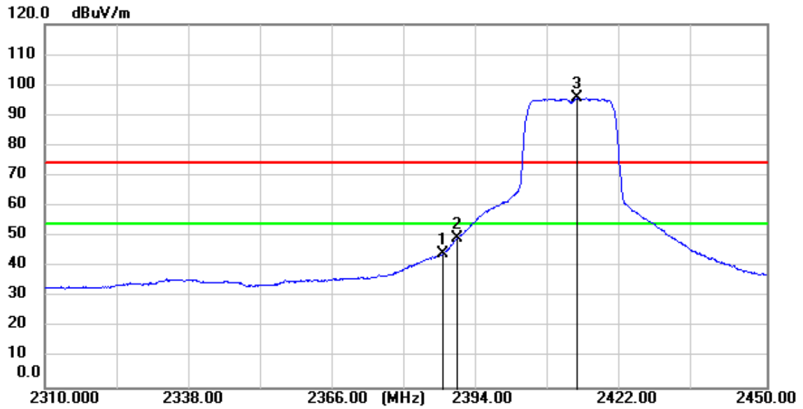
11n(HT20)_TX_CH_01_Vertical_Average
