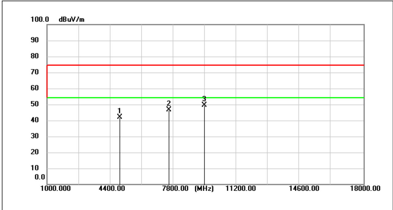
11b_TX_CH_11_Vertical
