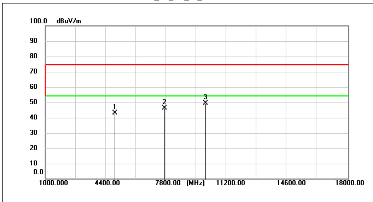
11b_TX_CH_11_Horizontal
