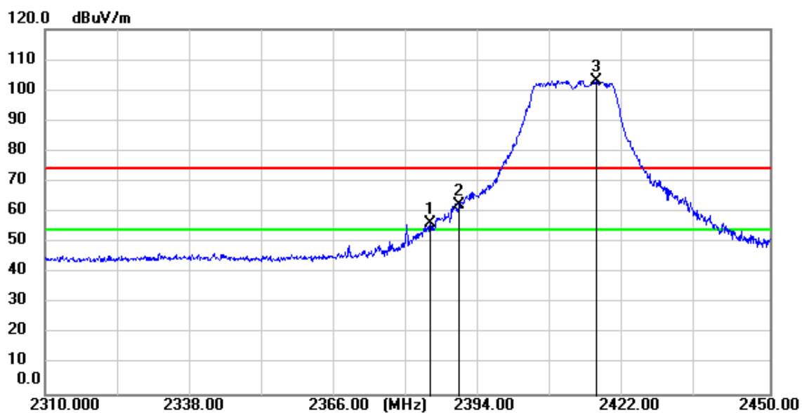
11n(HT20)_TX_CH_01_Horizontal_Peak
