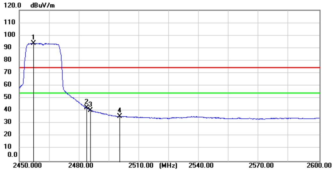
11n(HT20)_TX_CH_11_Vertical_Average
