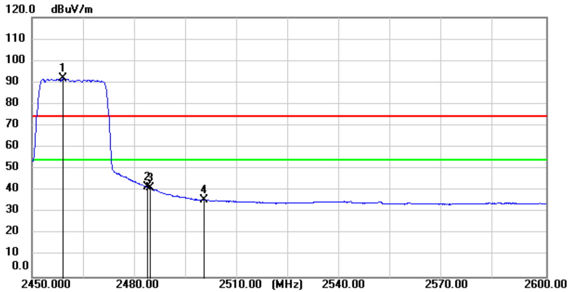
11(HE20)_TX_CH_11_Vertical_Average
