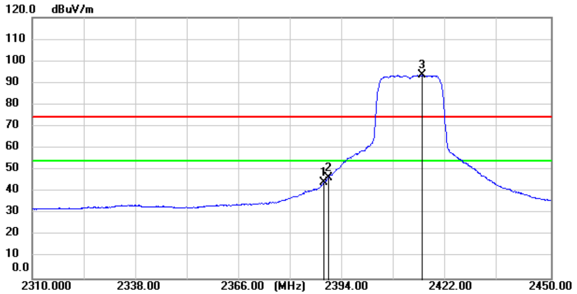
11n(HT20)_TX_CH_01_Horizontal_Average
