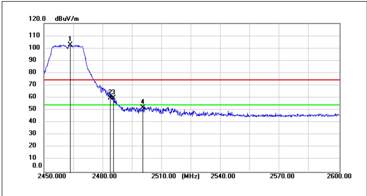
11n(HT20)_TX_CH_11_Horizontal_Peak
