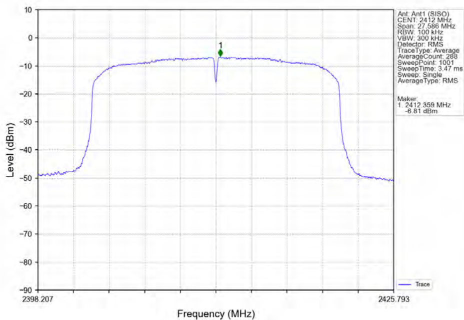
802.11ax(HE20) LCH 2412MHz SU / Ant1 (SISO) NTN
