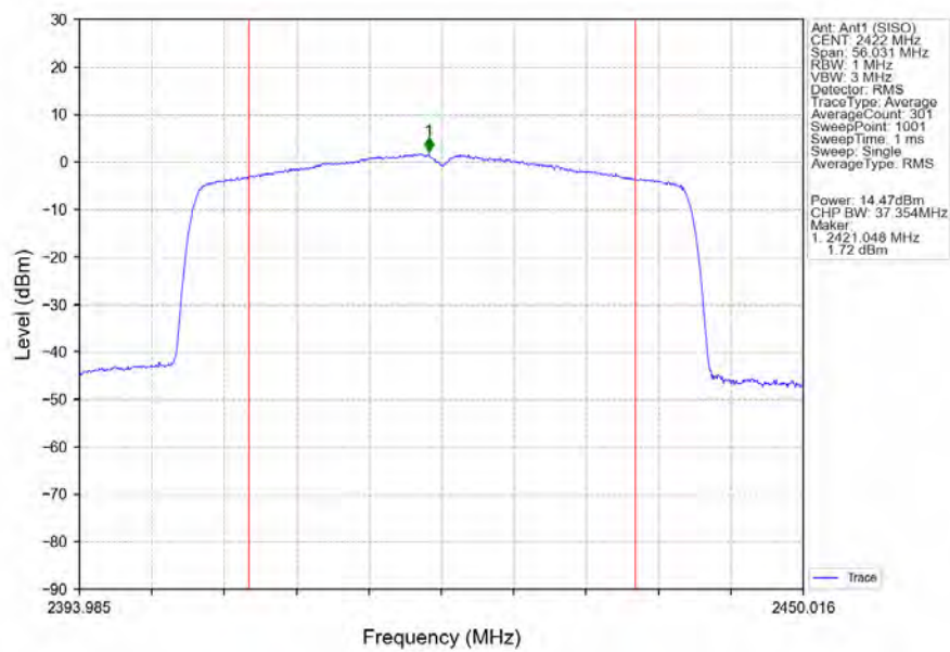
802.11ax(HE40) LCH 2422MHz SU / Ant1 (SISO) NTVN
