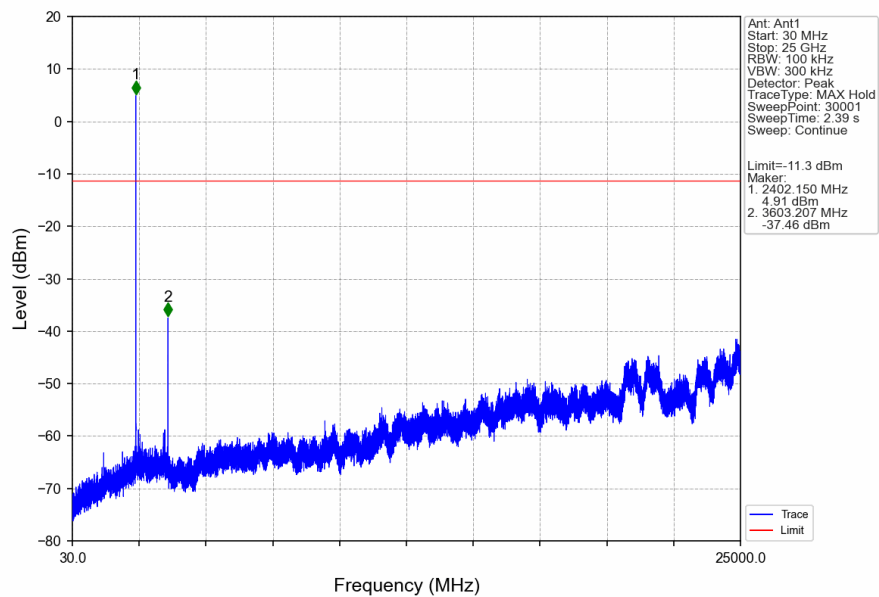
1M LCH 2402MHz Ant1 NTNV
