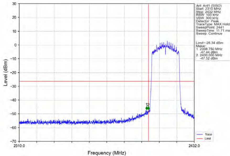
802.11ax(HE20) LCH 2412MHz SU / Ant1 (SISO) NTNV
