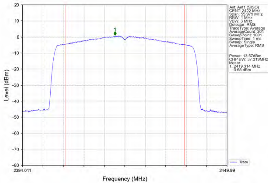
802.11ax(HE40) LCH 2422MHz SU / Ant1 (SISO) NTN
