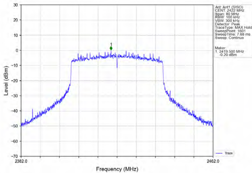
802.11ax(HE40) LCH 2422MHz_SU / Ant1 (SISO) NTV
