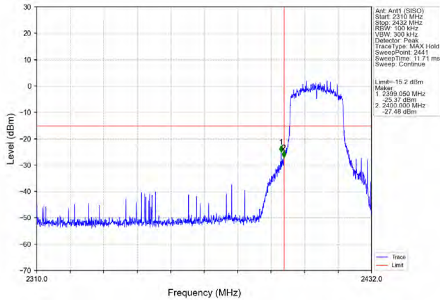
802.11ax(HE20) LCH 2412MHz SU / Ant1 (SISO) NTN
