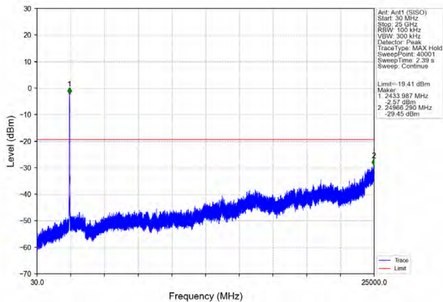
802.11ax(HE40) MCH_2437MHz_SU / Ant1 (SISO)_NTNV
