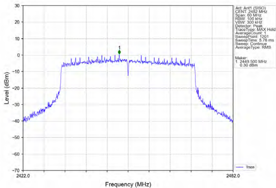
802.11ax(HE40) HCH 2452MHz SU / Ant1 (SISO) NTN
