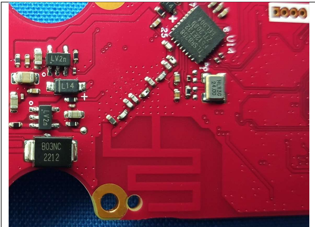
BLE Antenna
