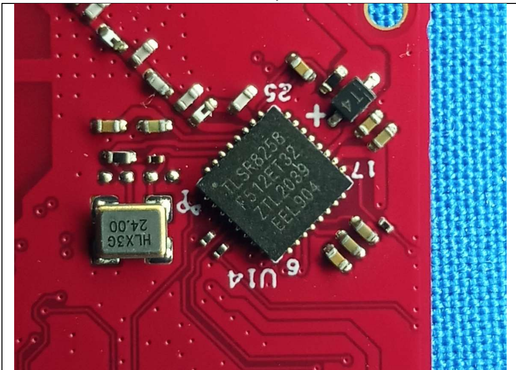
BLE Chip
