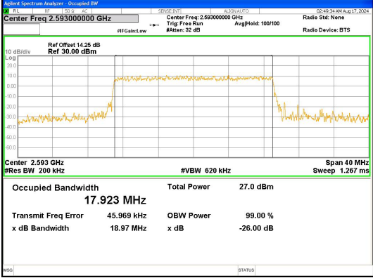
Band 41 20MHz/2593.0/Mid 16QAM 100@0
