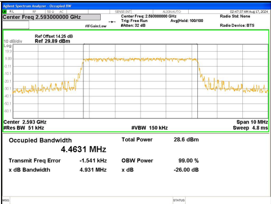
Band 41 5MHz/2593.0/Mid QPSK 25@0
