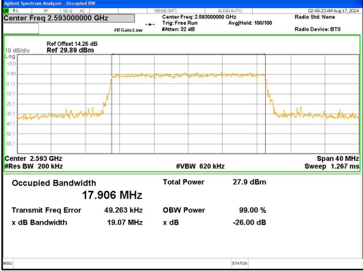
Band 41 20MHz/2593.0/Mid QPSK 100@0
