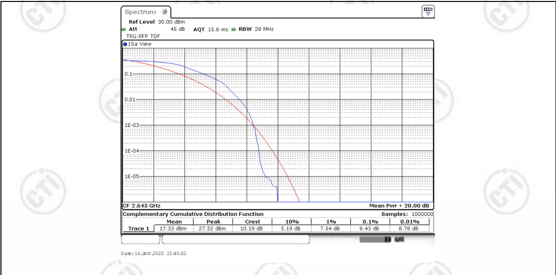
Band41-20MHz-QPSK-41140-1RB#0
