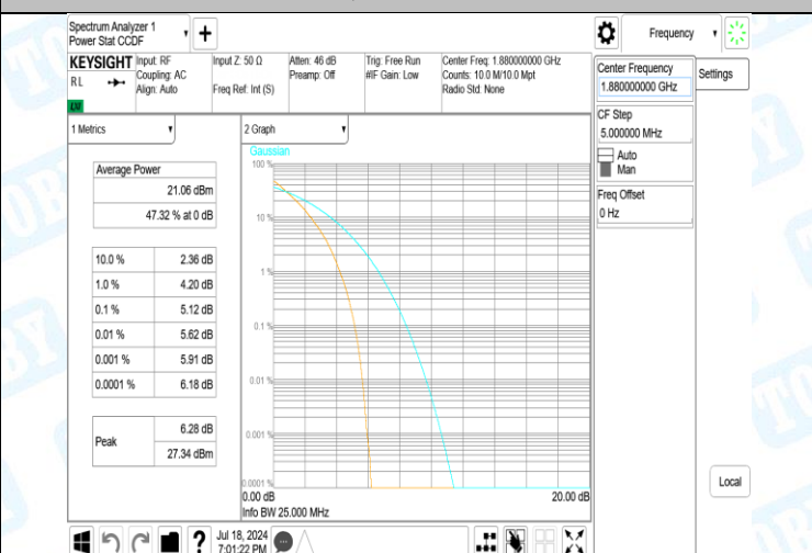
Band2-20MHz-QPSK-19100-100RB#0-PASS
