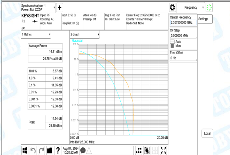
40(2350-2360)-10MHz-QPSK-39200-1RB#0-PASS
