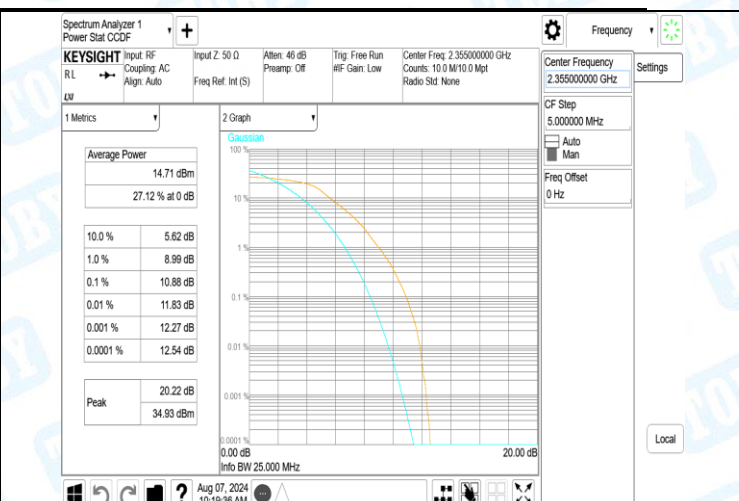
40(2350-2360)-5MHz-QPSK-39225-25RB#0-PASS
