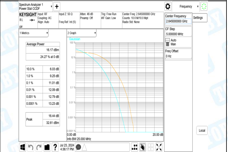
41(2555-2655)-20MHz-16QAM-41140-100RB#0-PASS
