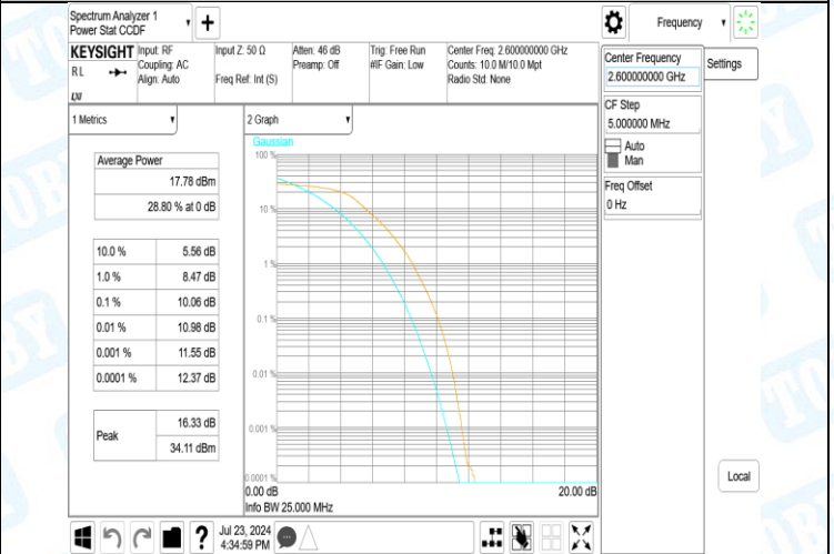
41(2555-2655)-20MHz-QPSK-41140-100RB#0-PASS
