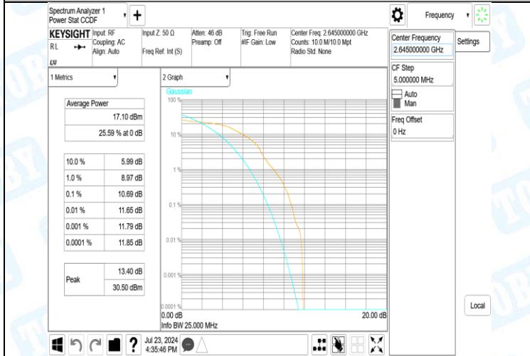
41(2555-2655)-20MHz-16QAM-41140-1RB#0-PASS
