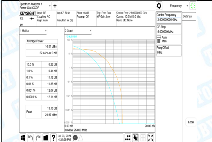
41(2555-2655)-20MHz-QPSK-41140-1RB#0-PASS
