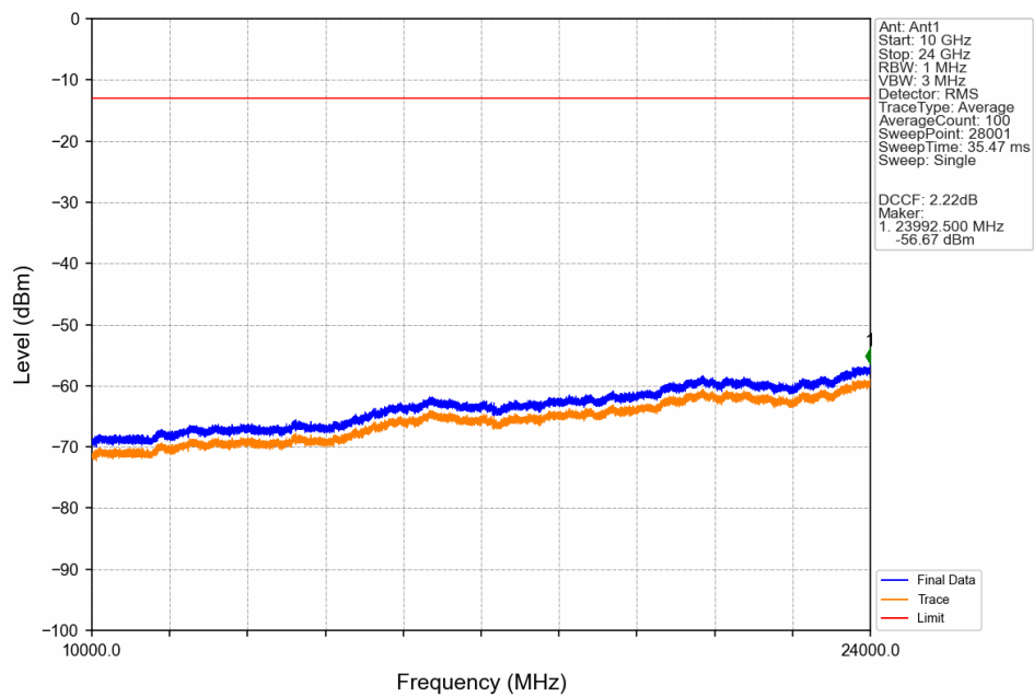
Band40_20MHz_QPSK_HCH_2390MHz_RB_1_0_NTNV
