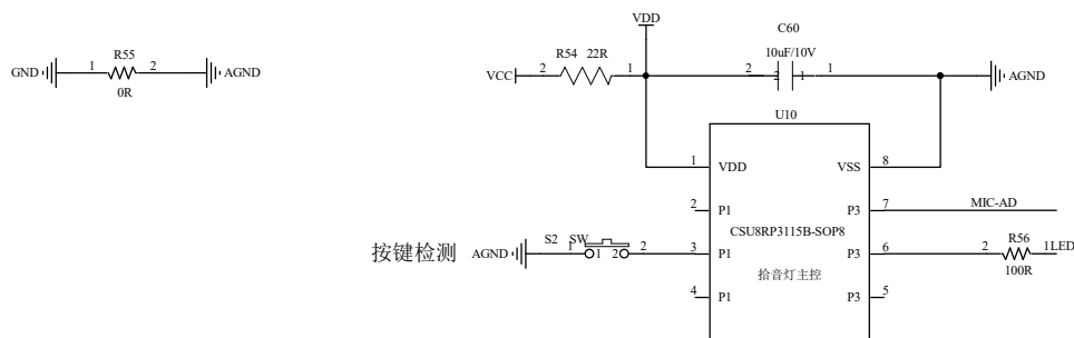
MCU控制电路
