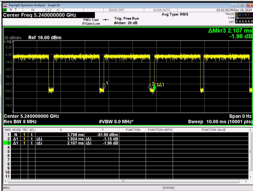
IEEE 802.11n_20MHz_Channel 48
