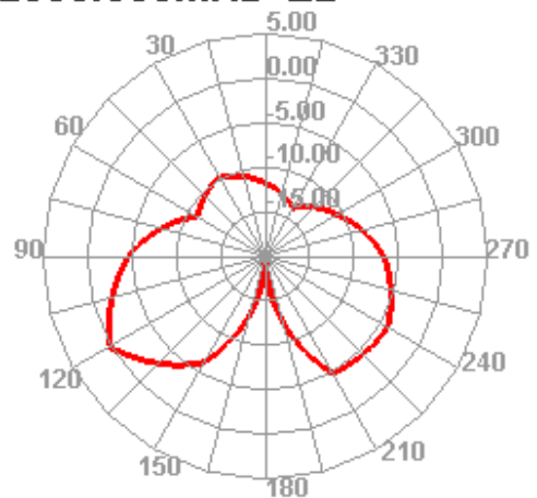
2500.000MHz E2
