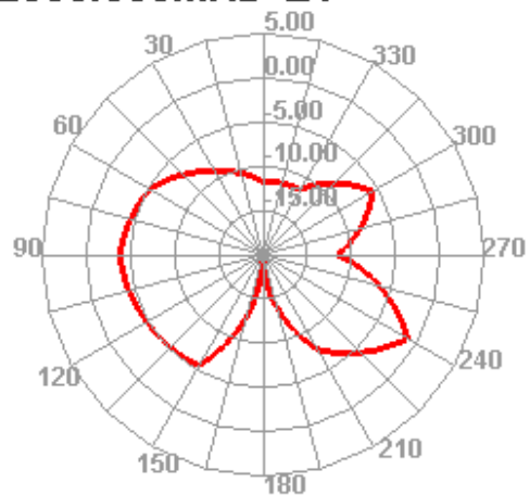
2500.000MHz E1
