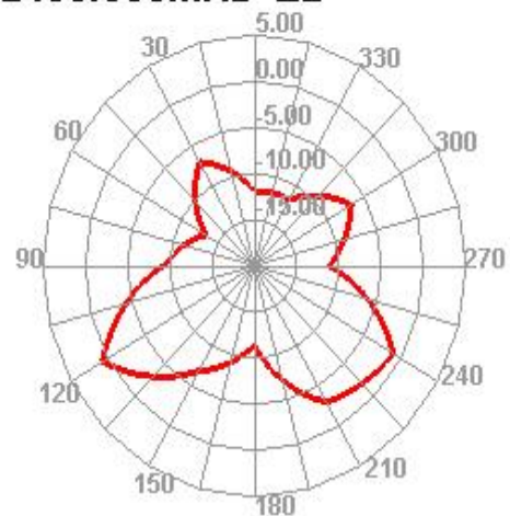
2450.000MHz H
