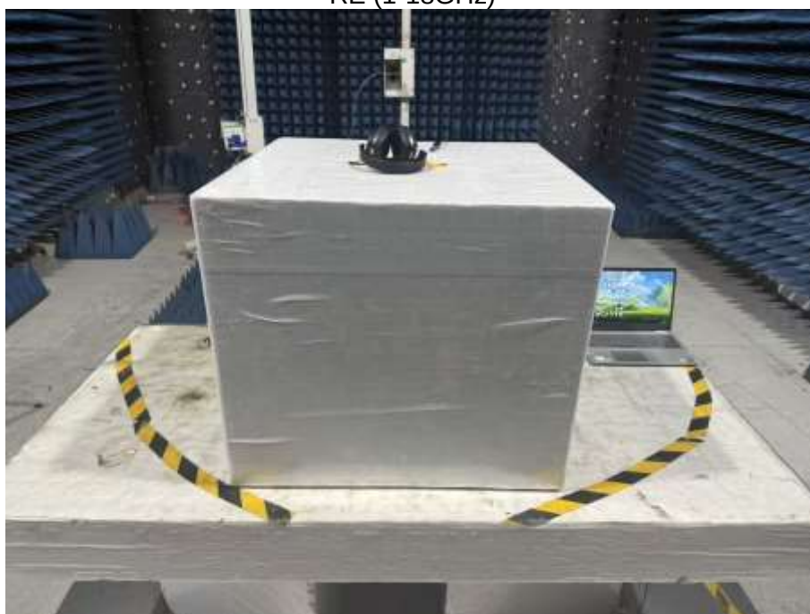
RE (1-18GHz)
