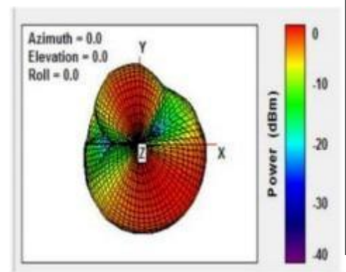
RadiatXion Pattern
