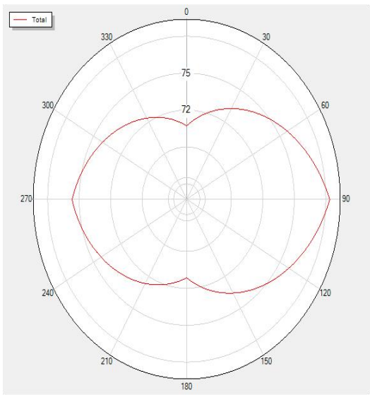
BLUETOOTH_Tis_Rssi_H0 Total
