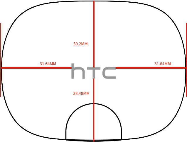
顶部 丝印
