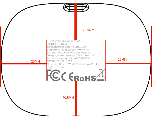
底部 丝印
