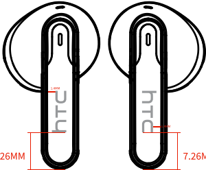
耳机正面 丝印
