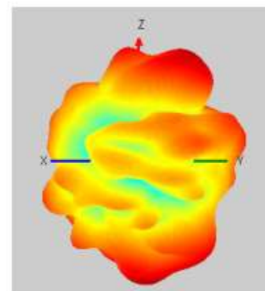
3D场形图
