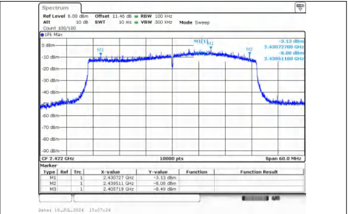
IEEE 802.11ax_Channel 3_40MHz_Antenna 1_RU&Index SU
