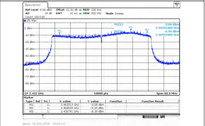
IEEE 802.11ax_Channel 9_40MHz_Antenna 1_RU&Index SU
