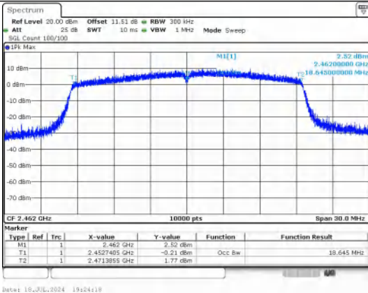
IEEE 802.11ax_Channel 11_20MHz_Antenna 1_RU&Index SU
