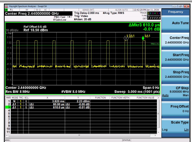
NTNV-2.4G SRD-Ant1-2440
