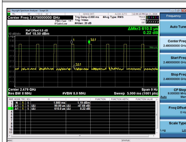
NTNV-2.4G SRD-Ant1-2479
