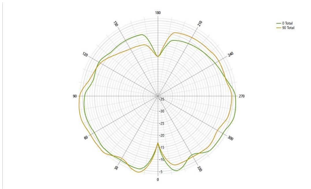
Phi=0°&Phi=90°_2500MHz
