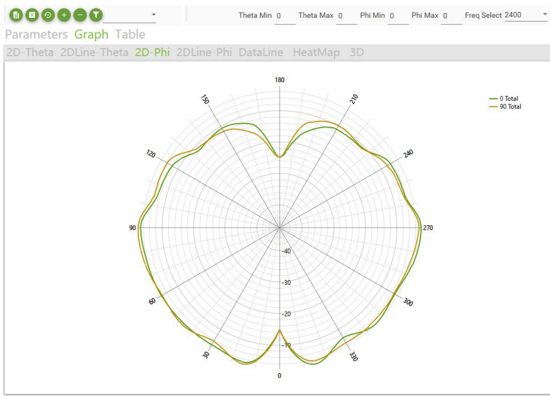
Phi=0°&Phi=90°_2400MHz
