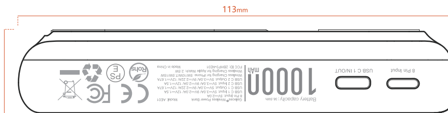
右视图 RIGHT
