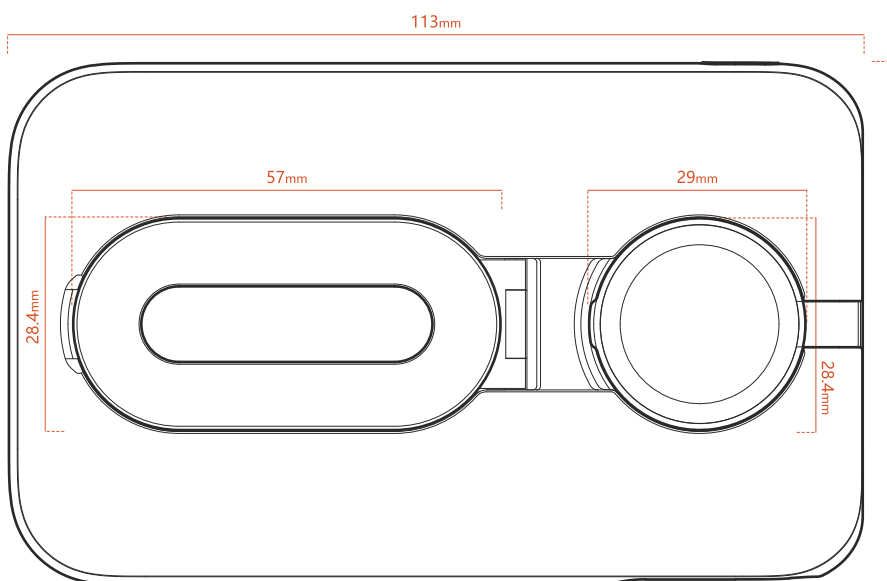
后视图 BACK
