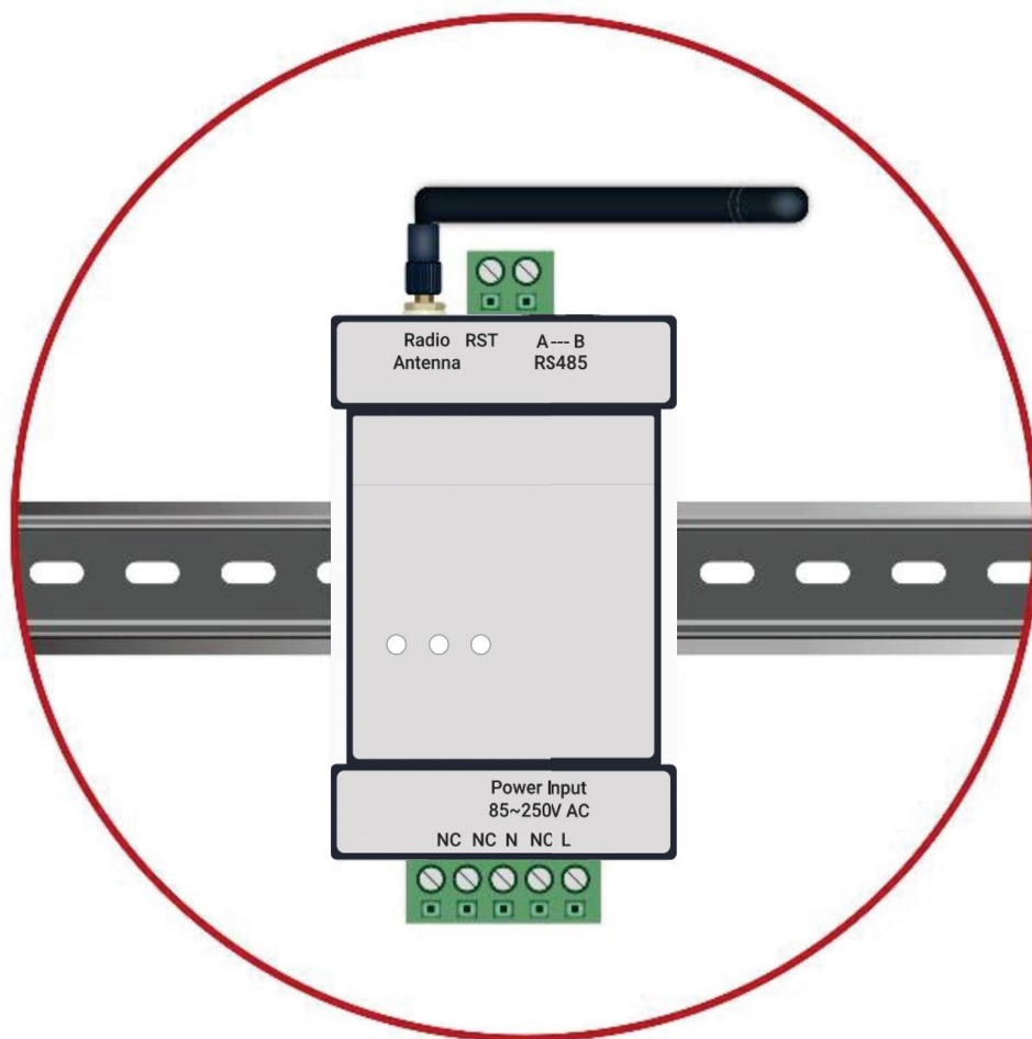
DIN rail installation
