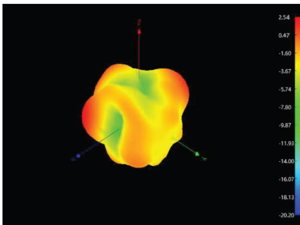
2480MHz 3D
