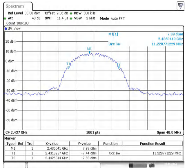
11B-Ant1-2437
