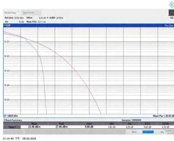
Band25-10MHz-16QAM-26365-1RB#0-PASS
