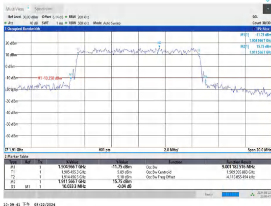
Band25-10MHz-QPSK-26640-50RB#0-PASS
