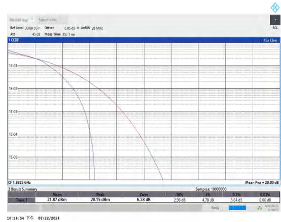
Band25-10MHz-16QAM-26365-50RB#0-PASS
