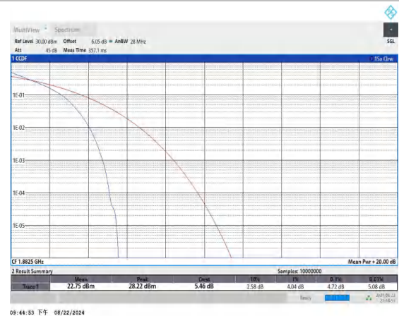
Band25-1.4MHz-QPSK-26365-6RB#0-PASS
