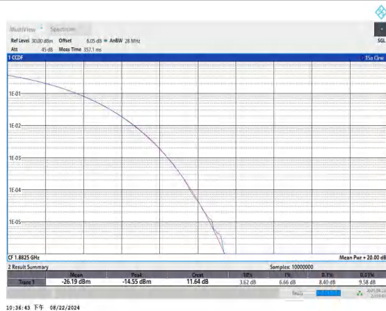
Band25-20MHz-16QAM-26365-1RB#0-PASS
