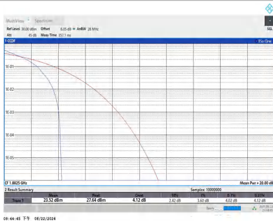
Band25-1.4MHz-QPSK-26365-1RB#0-PASS
