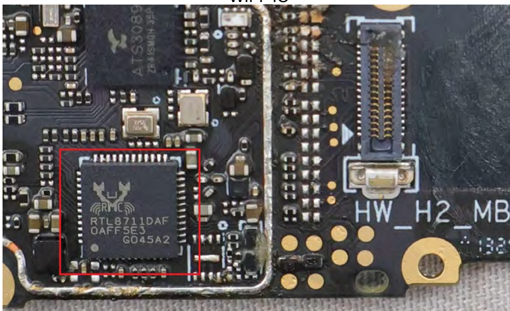
WIFI IC
