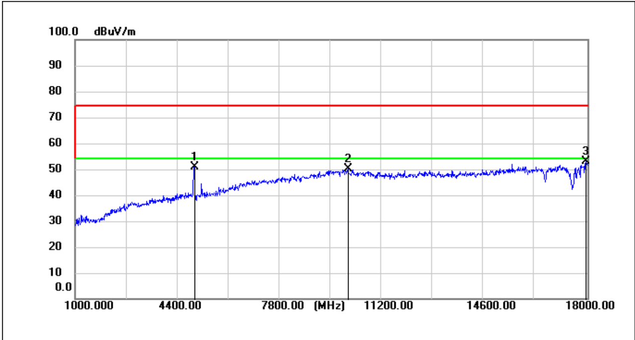
BLE_2M_TX_CH_39_Verical
