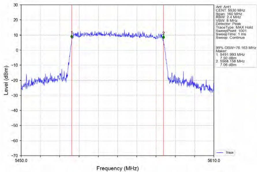
802.11ac(VHT80)_LCH_5530MHz_Ant1_NTNV
