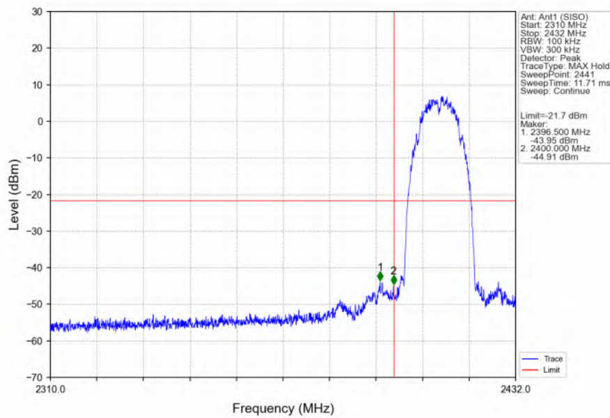
802.11b LCH 2412MHz_Ant1 (SISO)_NTNV
