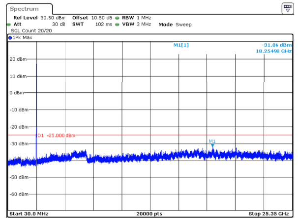
20MHz_Middle_QPSK_100@0
