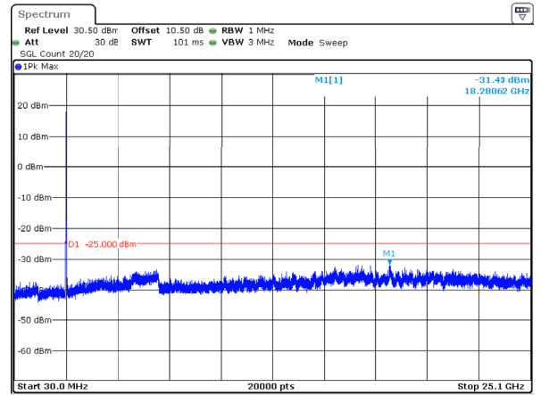
20MHz_Low_QPSK_100@0
