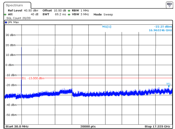
10MHz_Middle_QPSK_50@0
