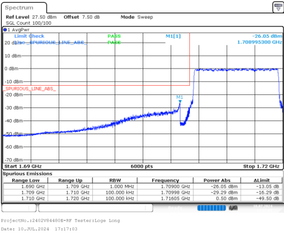
10MHz_Low_16QAM_50@0
