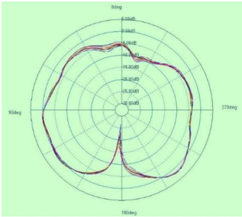
PHI=0
