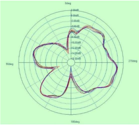
PHI=90
