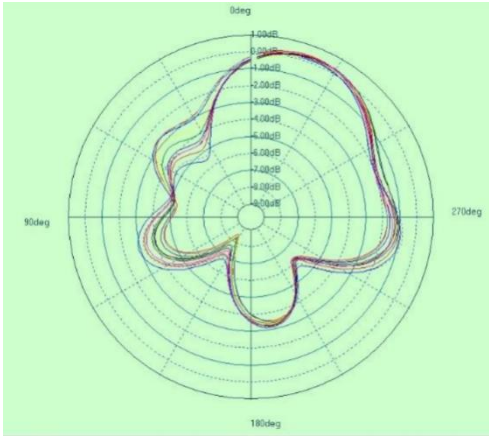
THETA=90
