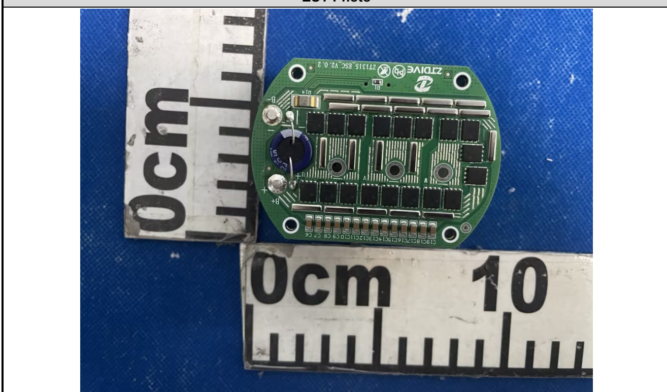
EUT Photo
