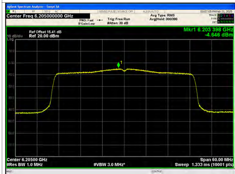
PSD NVNT ax40 6205MHz Ant1 SISO
