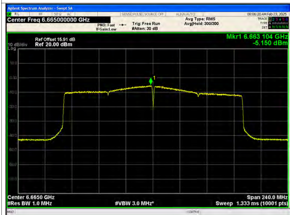
PSD NVNT ax160 6665MHz Ant2 MIMO
