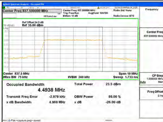
B19 / 5MHz / QPSK/ Mid CH
