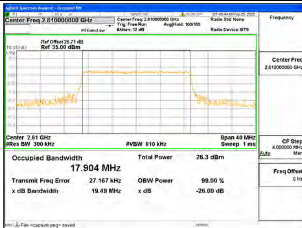
B38 / 20MHz / 64QAM/ High CH
