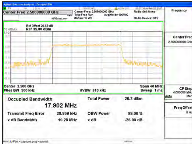
B41 / 20MHz / 64QAM/ Low CH
