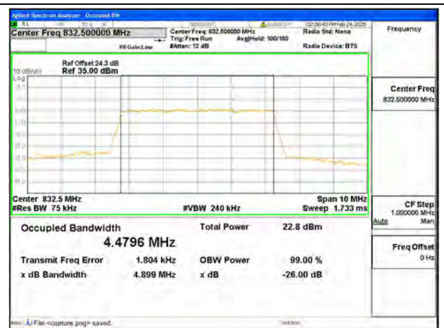
B19 / 5MHz / 16QAM/ Low CH
