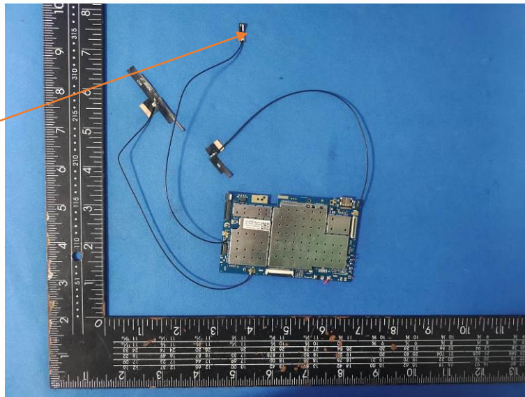
DIV ANT
