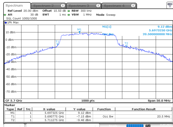
a_5700MHz_Chain 0
