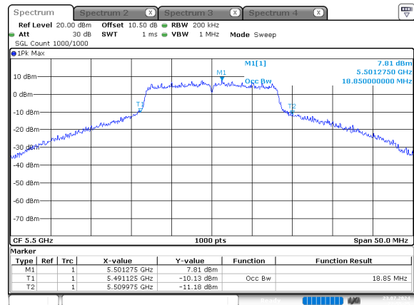
a_5500MHz_Chain 0
