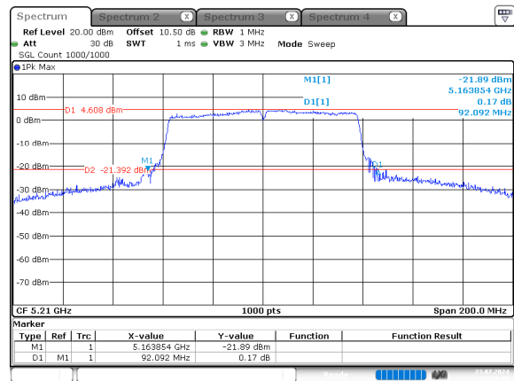
ac80_5210MHz_Chain 0
