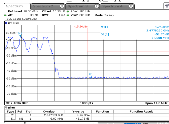
GFSK_Hopping_Upper
