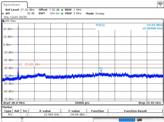
20MHz_Middle_QPSK_1@0
