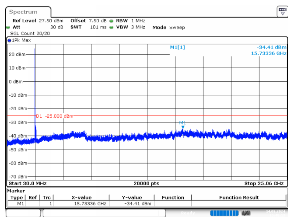
20MHz_Low_QPSK_1@0
